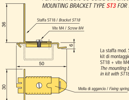
STAFFA DI FISSAGGIO MOD. ST3 - ACF000003 PER MONTAGGIO SU GUIDE DIN EN50022 MOUNTING BRACKET TYPE ST3 FOR DIN RAIL MOUNTING
